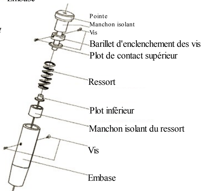
Tête de pointe de fleuret de type français
