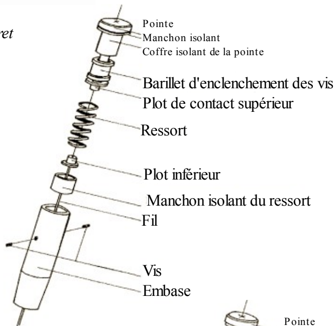
Tête de pointe de fleuret de type allemand
