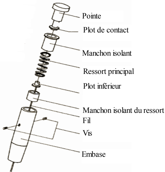
Tête de pointe de fleuret de type anglais
